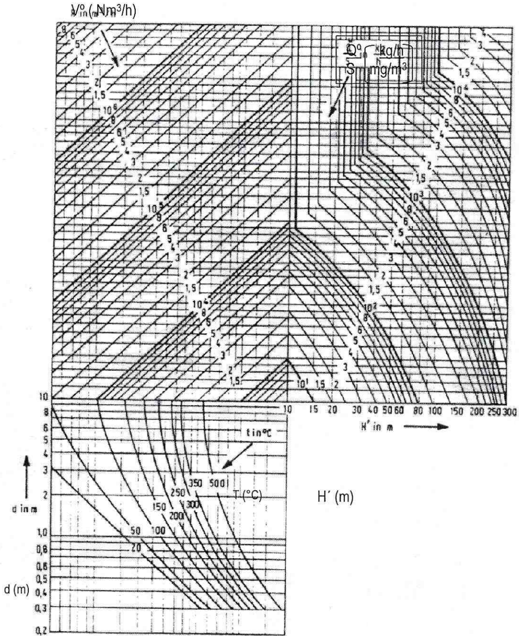
Gráfica 1. Nomograma para el cálculo de la altura mínima de chimenea.
