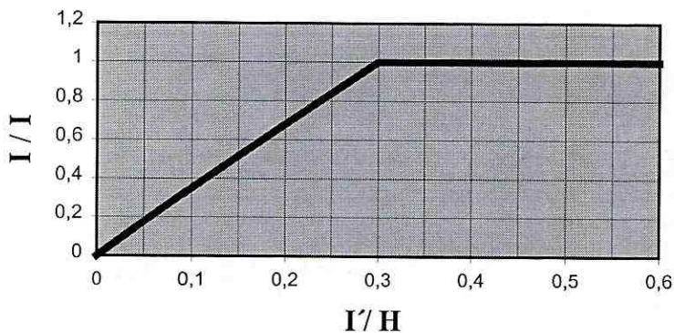
GRAFICA DE CORRECCION DE ALTURA
